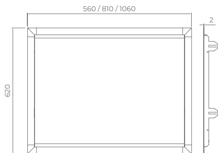
Marco a nivel para el armario Slim
