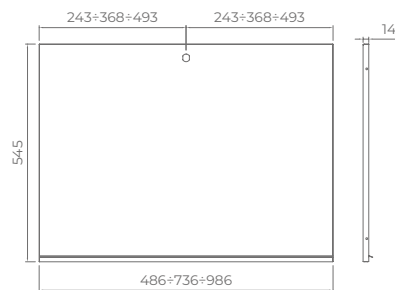
Puerta para armario Slim
